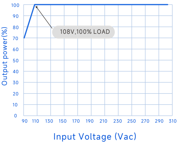
降额曲线（输出功率Vs.输入电压）
